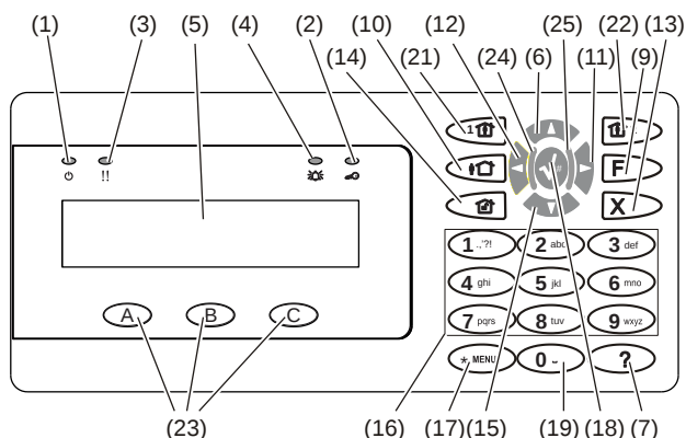
Ábra 2: ATS1135 kezelő
